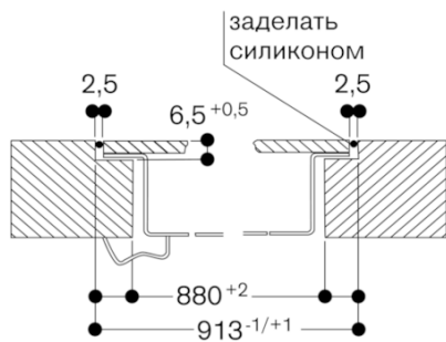
Продольный разрез
